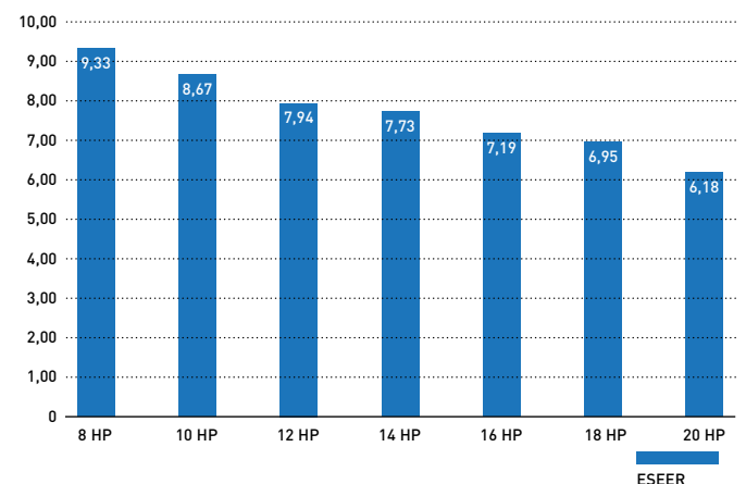
ESEER (W/W)
